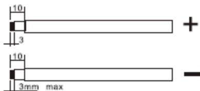
Рисунок 5 Разделка солнечного кабеля
